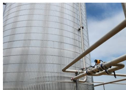
음성가축분뇨처리장 바이오가스 소화조125A, 발전기125A 라인 FN질량유량계
