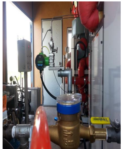
보일러 Water공급, 50A 라인 FN질량유량계
