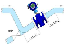
곡선 파이프 하향 경사 상향 배관 설치 방법
