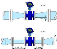
샤프트 파이프 및 확장 파이프 설치 방법
