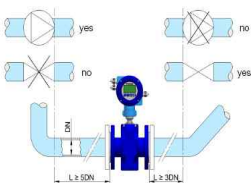
곡선 파이프 하향 수평 배관 설치 방법
