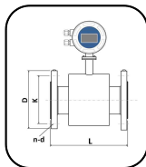
인라인 일체형 KC-8860-M
