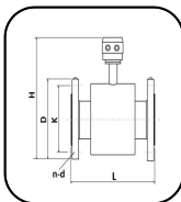
인라인 컨버터 분리형 KC-8860-D
