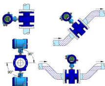
파이프 종류별 유량 설치 방법
